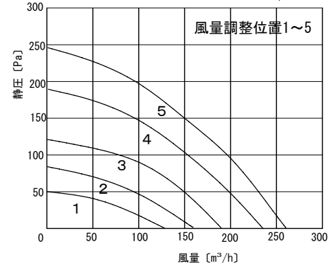
静圧-風量特性曲線 50/60Hz
